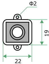
【上面図】
